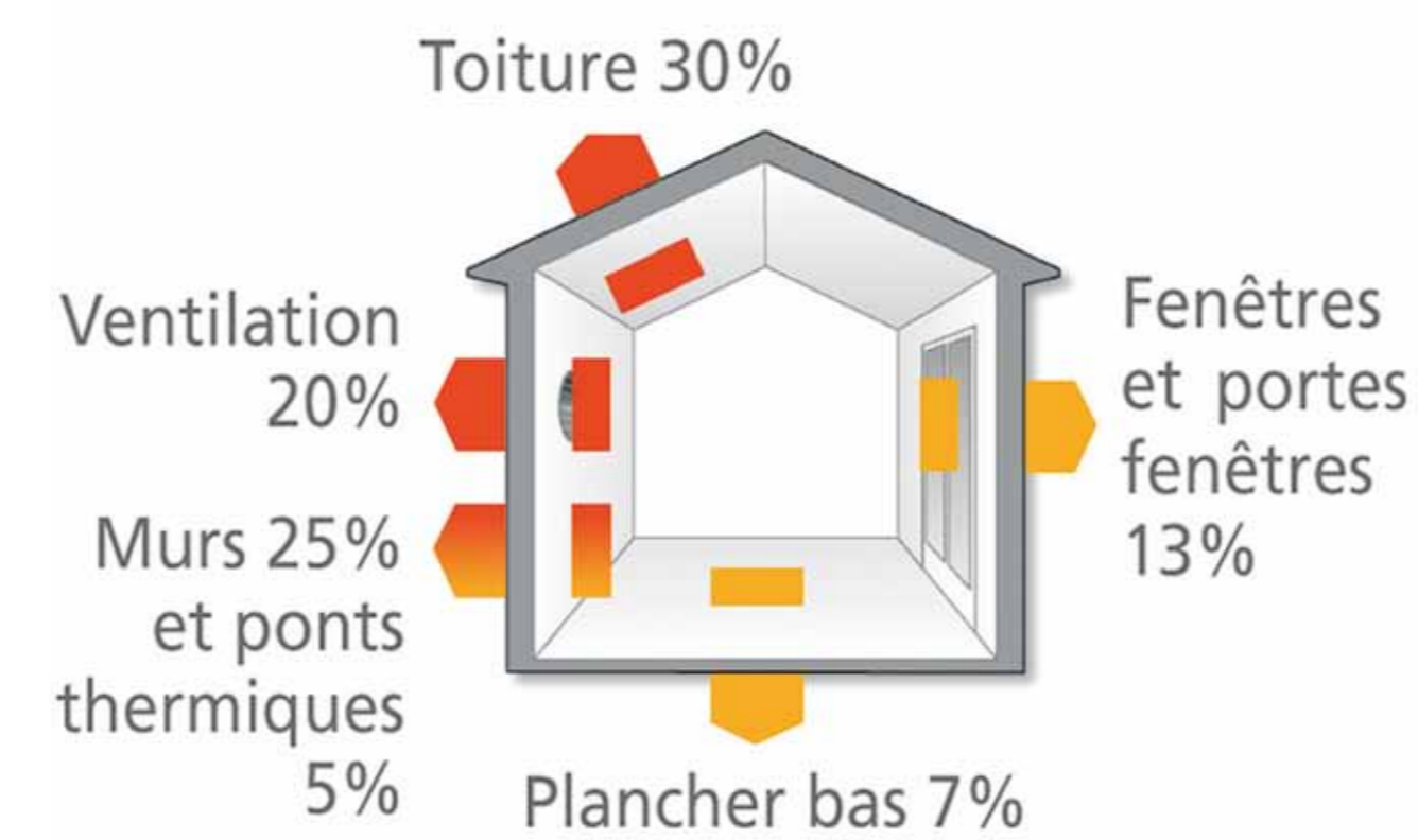
Déperditions de chaleur d'une maison mal isolée
